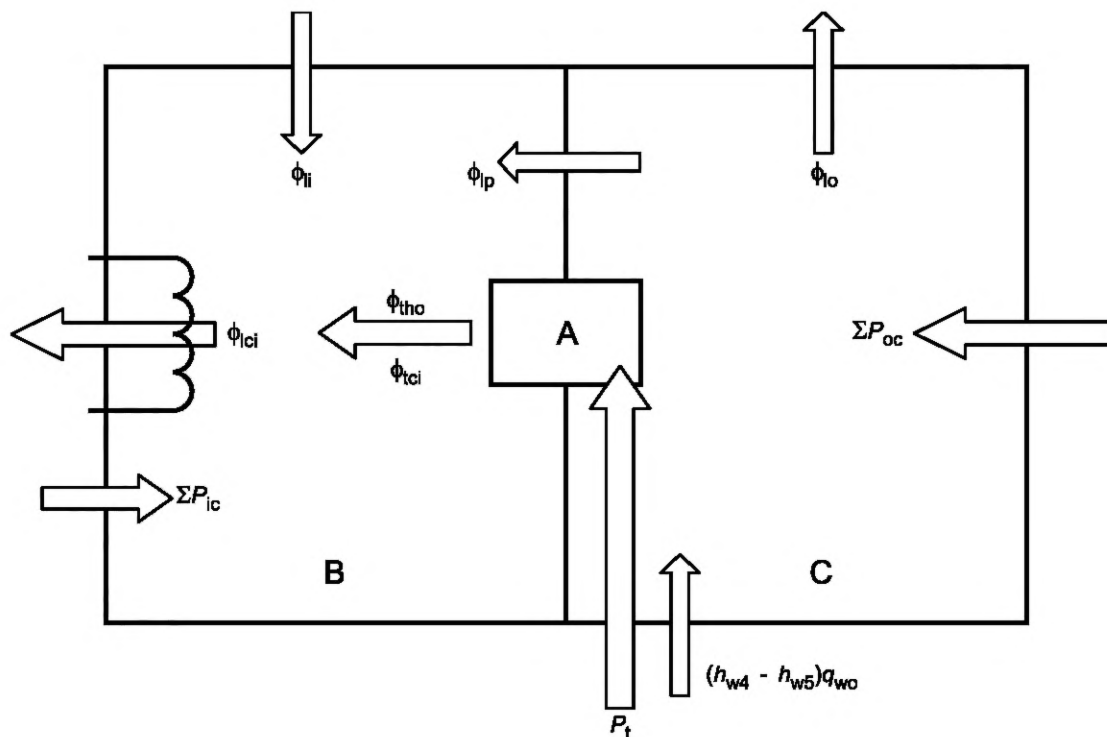
Рисунок А.4 — Поток энергии в калориметрической установке во время испытаний теплопроизводительности
