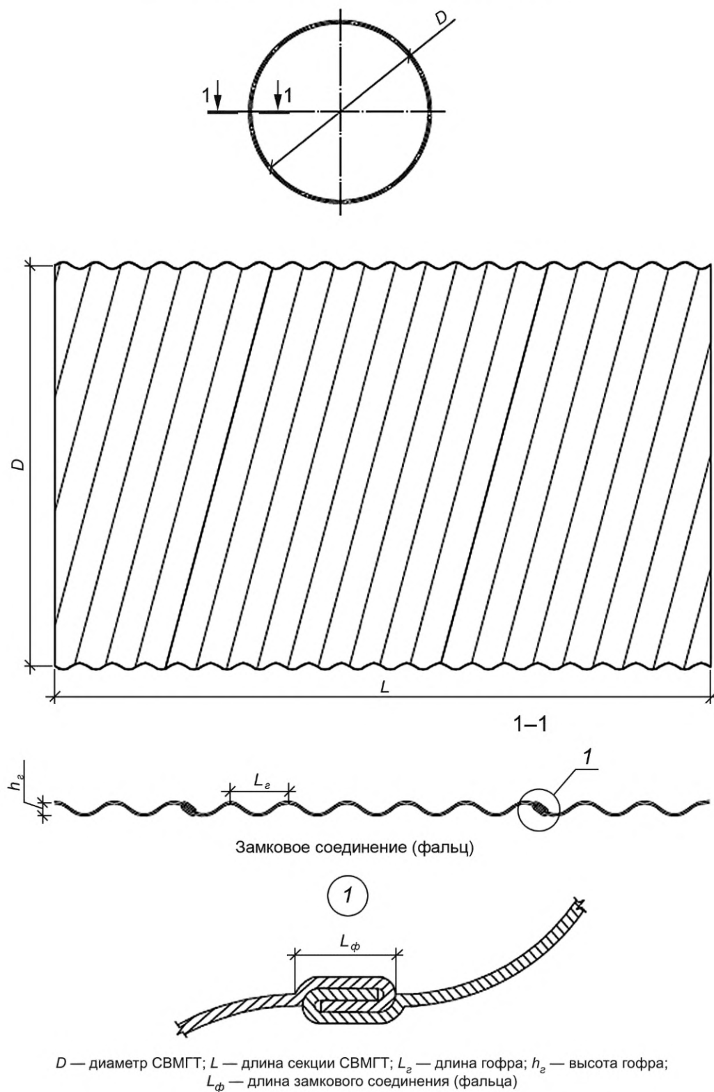
Рисунок А.1 — Конфигурация и геометрические размеры СВМГТ
