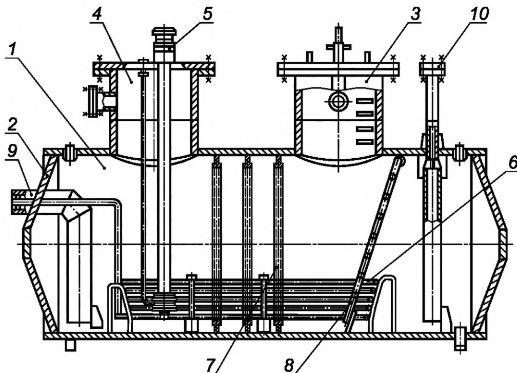
1 — обечайка; 2 — днище; 3 — люк-лаз; 4 — люк насосного агрегата; 5 — насосный агрегат; 6 — подогреватель; 7 — кольцо жесткости; 8 — лестница; 9 — патрубок; 10 — штуцер уровнемера
