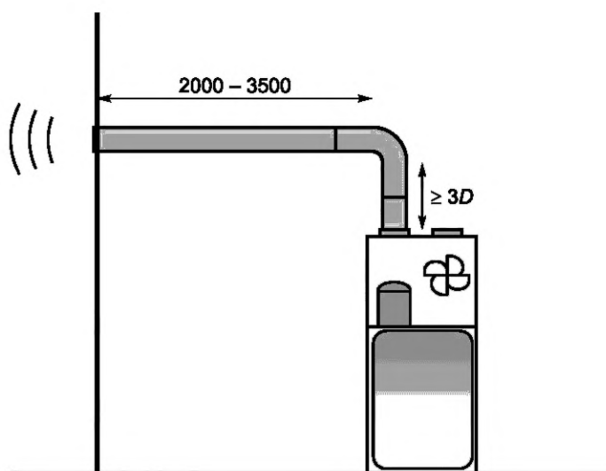
Рисунок 1 — Длина воздуховода
