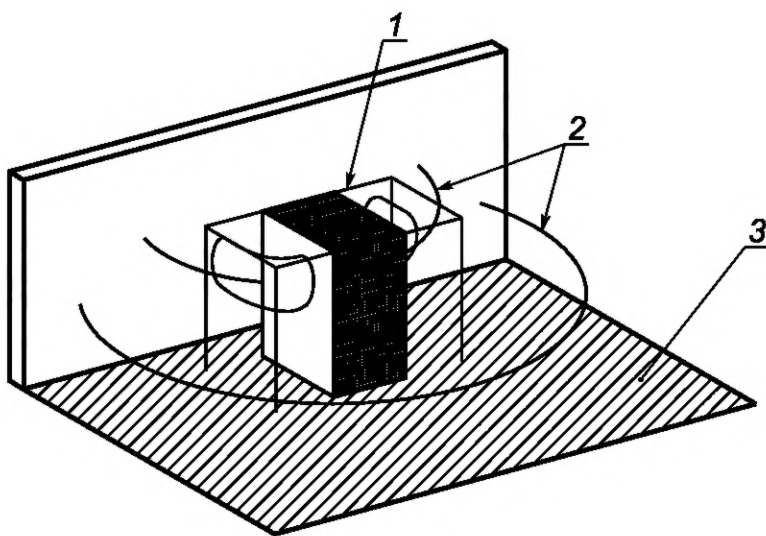
Рисунок 6 — Измерение уровня звуковой мощности L_{Wio} с использованием метода свободного звукового поля над звукоотражающей плоскостью
