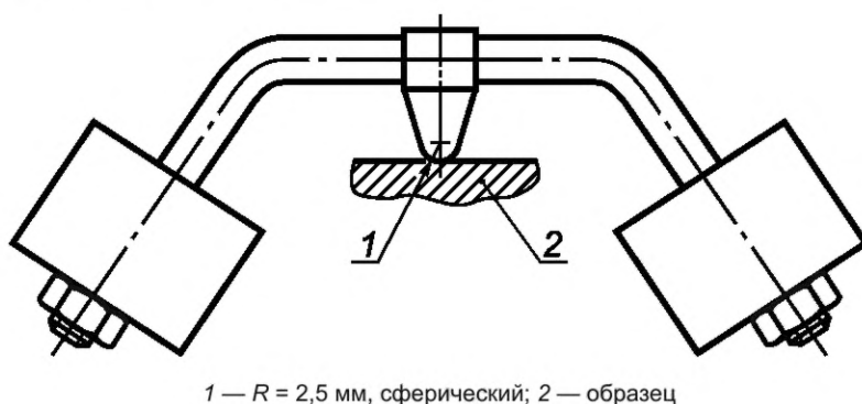
Рисунок 10 — Устройство для испытания давлением шарика
