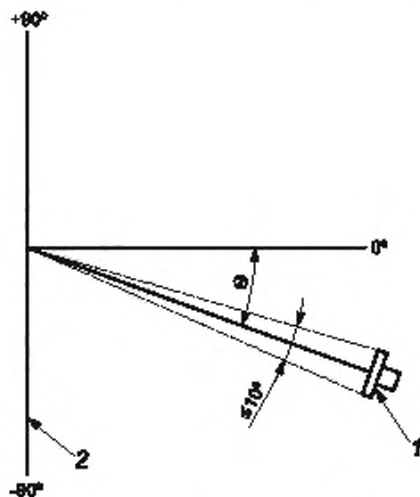
1 — радиометр; 2 — передняя поверхность системы диффузного освещения
