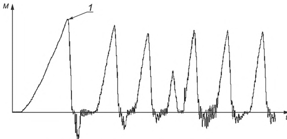
Рисунок 109 — Пример крутящего момента машины без стабильной области сигнала
