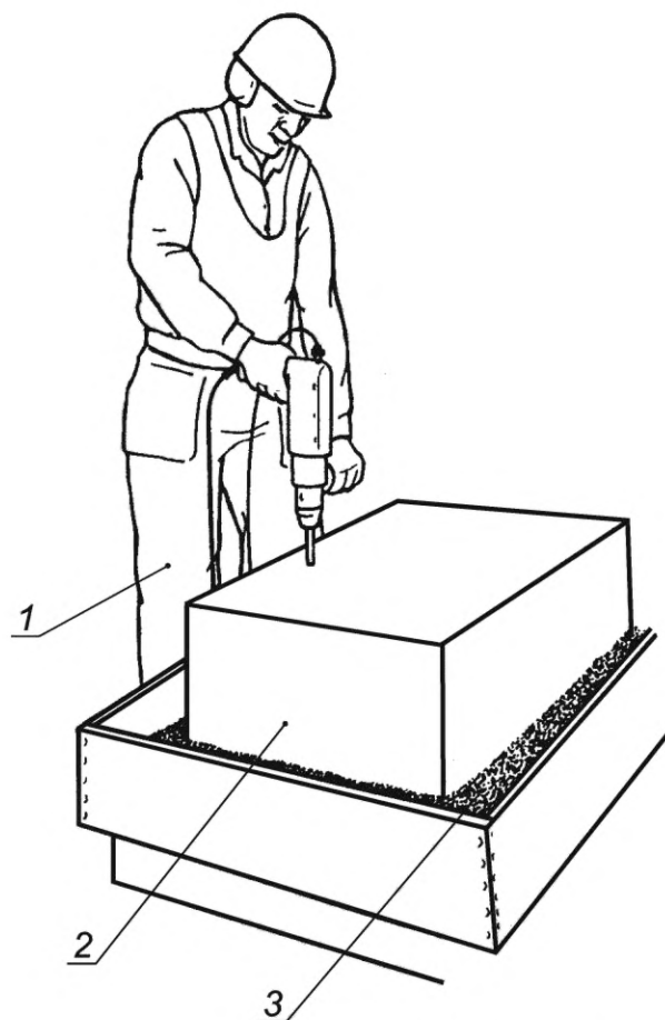
Рисунок I.101 — Применение нагрузки
