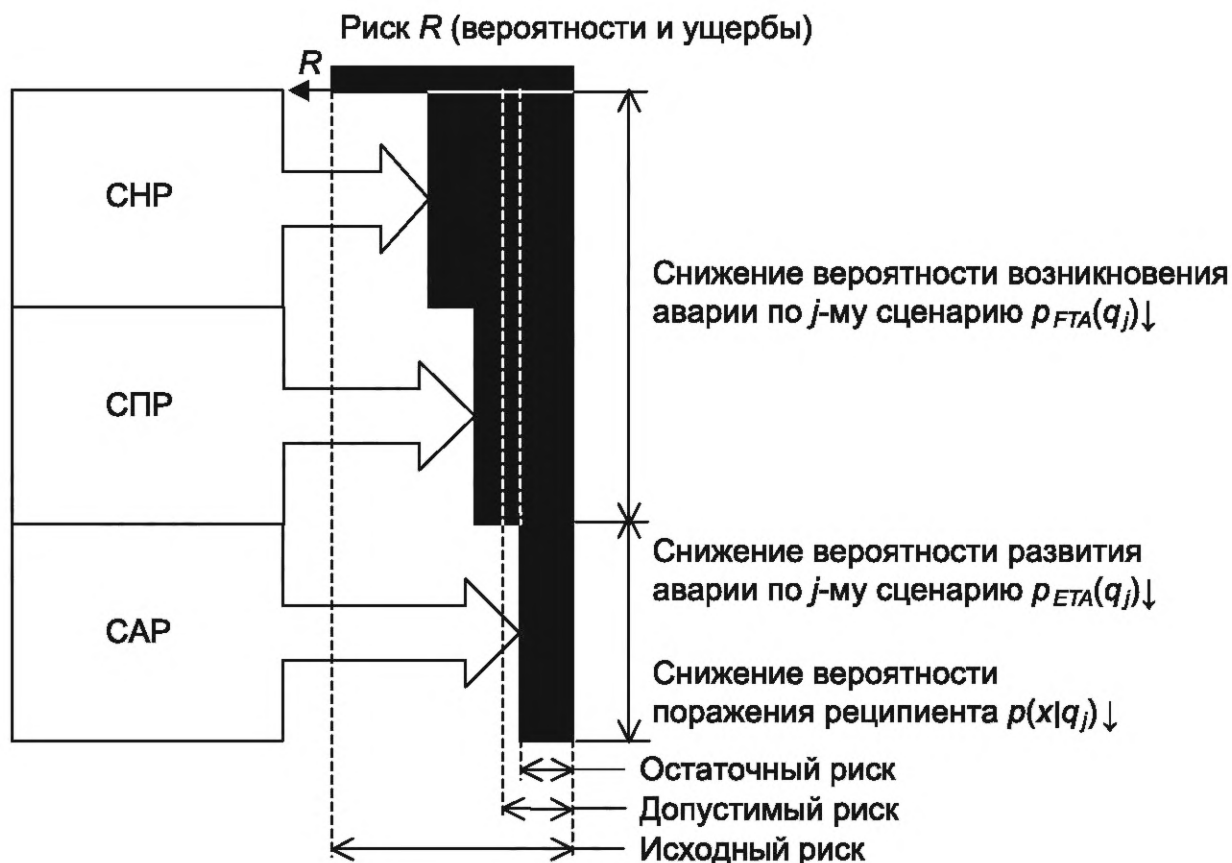
Рисунок 5 — Снижения риска с помощью МФСБ
