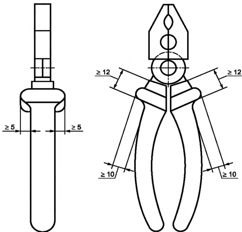
Рисунок 8 — Изоляция плоскогубцев
