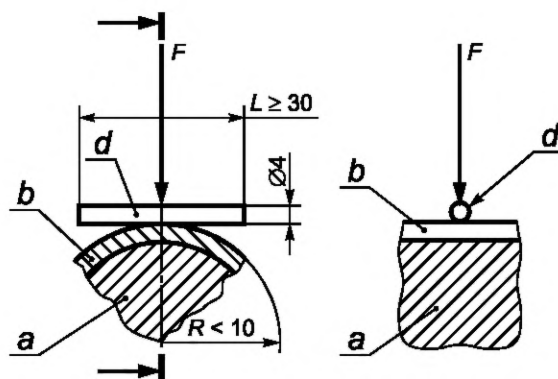
Рисунок 20b — Радиус в контрольной точке инструмента < 10 мм
