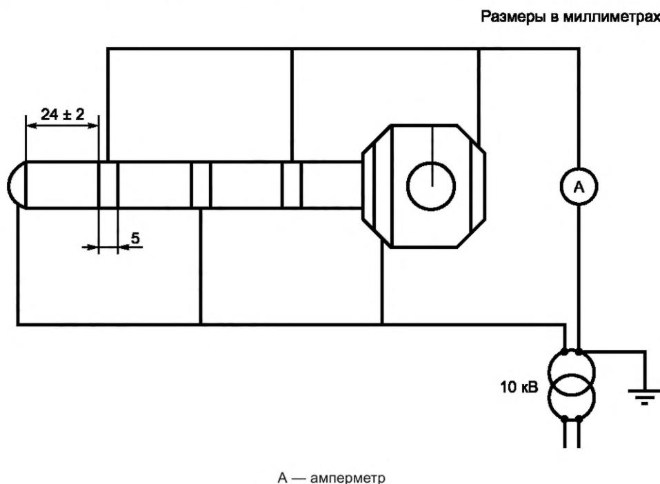
Рисунок 19 — Схема испытания электрической прочности изоляции изолирующих инструментов
