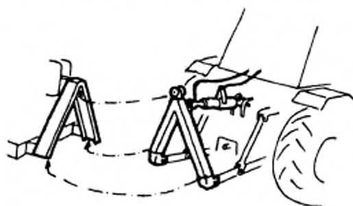
Рисунок 1 — Принцип работы системы с А-образным сцепным устройством
