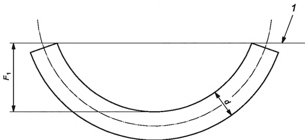
Рисунок 2 — Определение прогиба F_1
