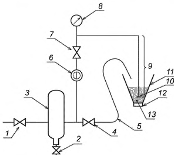
1 — клапан А, 2 — клапан В, 3 — фильтр, 4 — клапан С; 5 — резиновый шланг; 6 — клапан контроля давления воды; 7 — клапан D; 8 — манометр, 9 — сопло; 10 — наконечник сопла; 11 — воронка, 12 — сито, 13 — технический углерод
