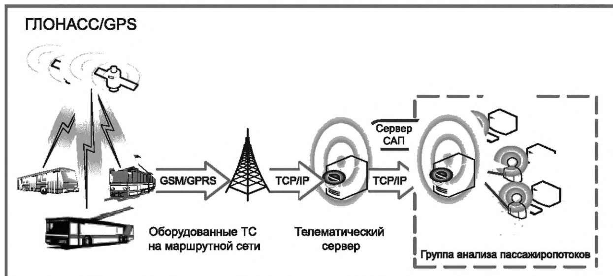
Рисунок 2 — Схематическое отображение процесса сбора и обработки информации в СПП
