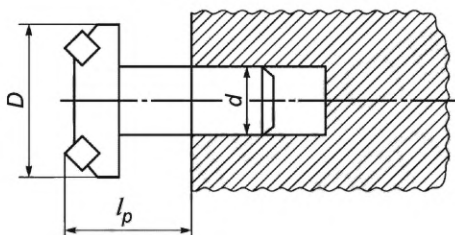
Рисунок 4 — Пример для сборной фрезы
