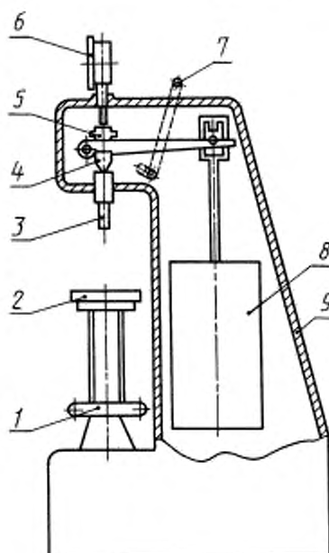
1 — гайка-маховик; 2 — подъемный столик; 3 — индентор; 4 — призма рычага основной нагрузки; 5 — шпиндель с грузом предварительной нагрузки; 6 — отсчетное устройство; 7 — рукоятка приложения и снятия основной нагрузки; 8 — грузы для основной нагрузки; 9 — корпус
