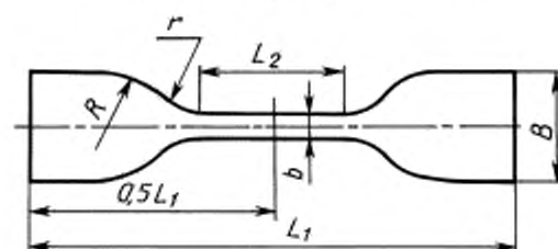
Рисунок 2 — Образец-лопатка типа 2
