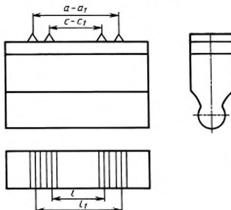
Схема штампа для нанесения меток на образец
