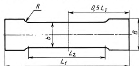
Рисунок 1 — Образец-лопатка типа 1
