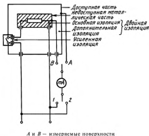
Рисунок 25 — Схема измерения тока утечки при рабочей температуре для однофазных устройств класса II
