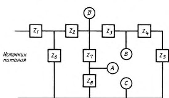
Рисунок Н.27.1.1 — Пример электронной цепи с маломощными точками
