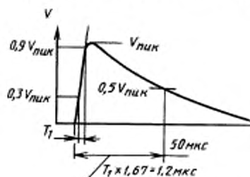
Рисунок Н.26.8.1 — Форма волны при разомкнутой цепи
