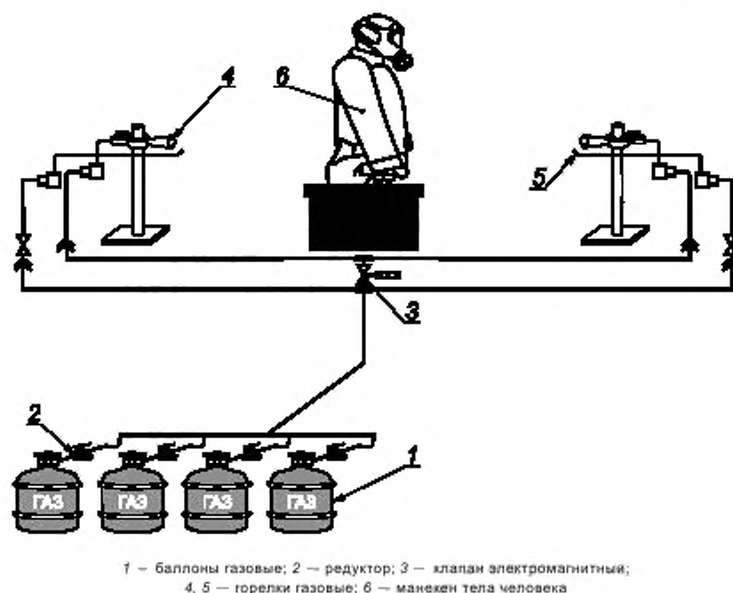
Рисунок А.1 — Схема стенда по определению устойчивости лицевой части к воздействию пламени
