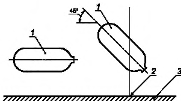
1 — испытываемый баллон; 2 — точка соударения; 3 — испытательная плита
