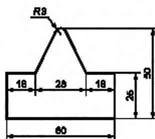
Рисунок 2 — Поперечный профиль и размеры бойка
