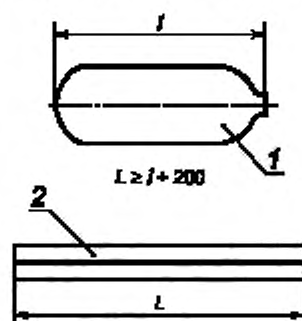
1 — испытываемый баллон; 2 — боек
