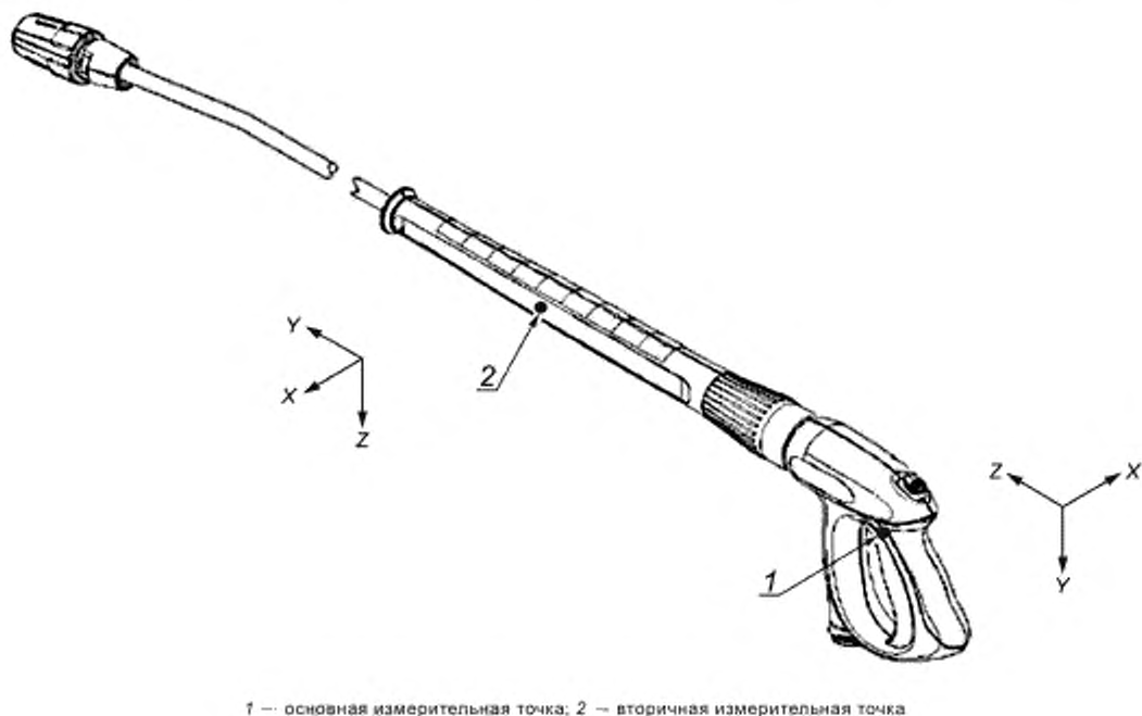
Рисунок DD.3 — Места расположения измерений: пистолет-распылитель, основная и вторичная измерительная точка
