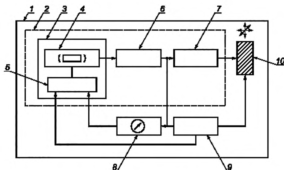
1 — лазерный блок; 2 — лазерная установка; 3 — лазерное устройство; 4 — лазер; 5 — подача (мощности, охлаждения, газа); 6 — устройство направления пучка (зеркала, волокна, линзы); 7 — устройство формирования пучка (телескоп, фокусировка); 8 — системы измерения и системы управления; 9 — блоки обработки (робот, обрабатываемый объект, его местоположение); 10 — обрабатываемый объект
