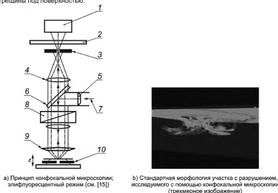
Рисунок 18 — Принцип конфокальной микроскопии
