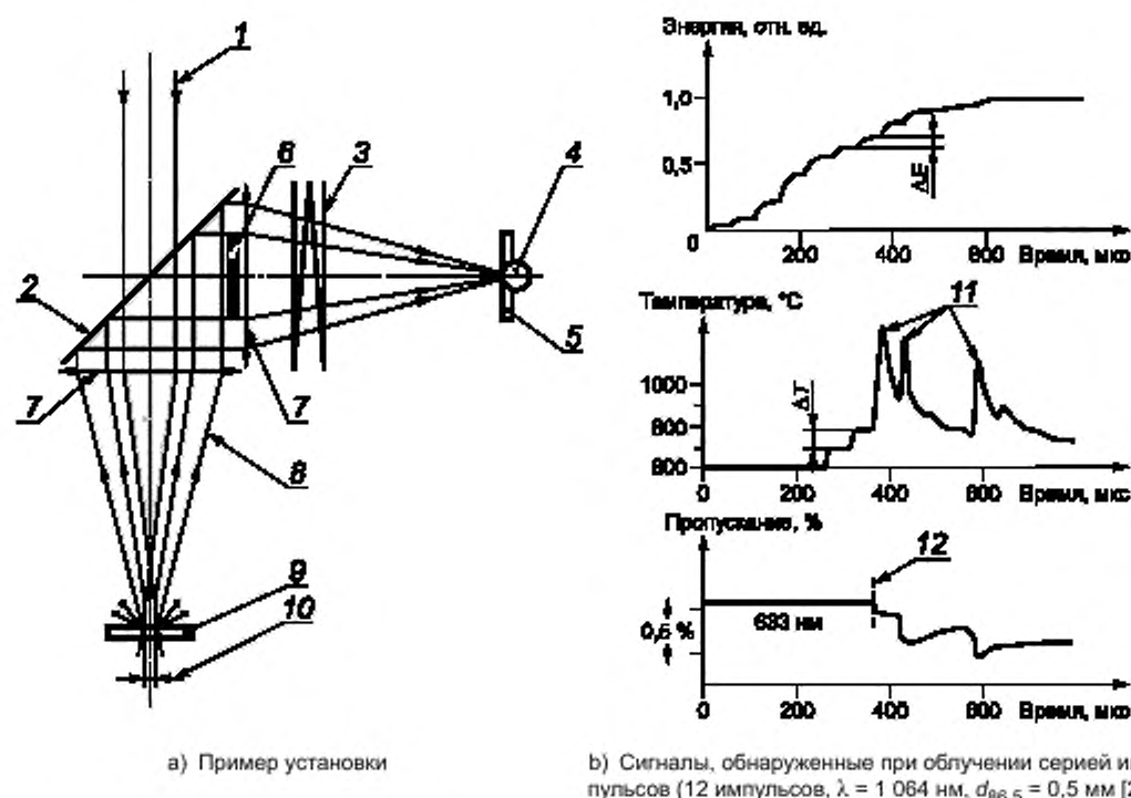
а) Пример установки б) Сигналы, обнаруженные при облучении серий импульсов (12 импульсов, \lambda = 1\,064\text{ нм} , d_{86,5} = 0,5\text{ мм} [2])
