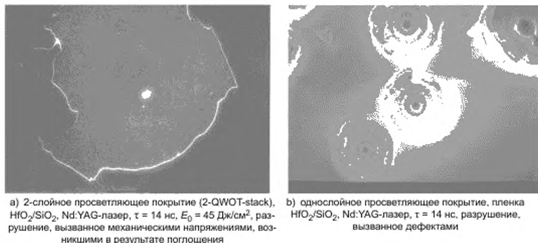
Рисунок 16 — Изображение, полученное при техническом осмотре: СЭМ-микроснимки различных участков с разрушением
