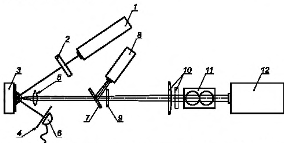
1 — гелий-неоновый лазер; 2 — затенитель; 3 — образец; 4 — микроотверстие; 5 — фокусирующая линза; 6 — фотодиод; 7 — светоделитель; 8 — пирометр; 9 — фотошаблон; 10 — гомогенизатор и полевая линза; 11 — переменный затенитель; 12 — эксимерный лазер
