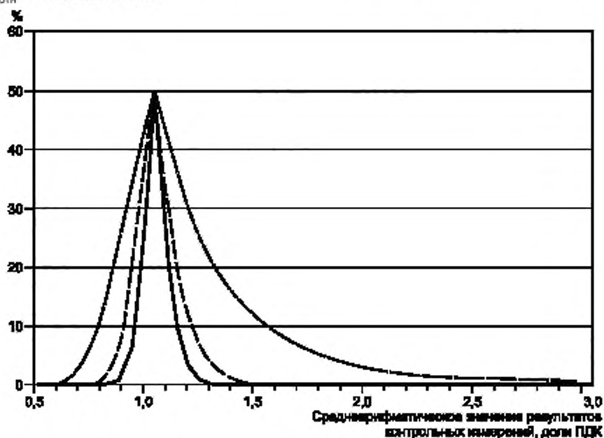
Рисунок 1 — Вероятность ложных заключений о качестве воды (ось ординат) при \delta_{изм} = 10\% . Сплошная линия соответствует \delta_{выб}/\delta_{изм} = 2 , штриховая — \delta_{выб}/\delta_{изм} = 4 , пунктирная — \delta_{выб}/\delta_{изм} = 10
