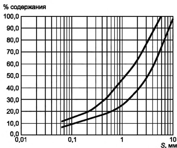
Рисунок 4 — Кривая гранулометрического состава
