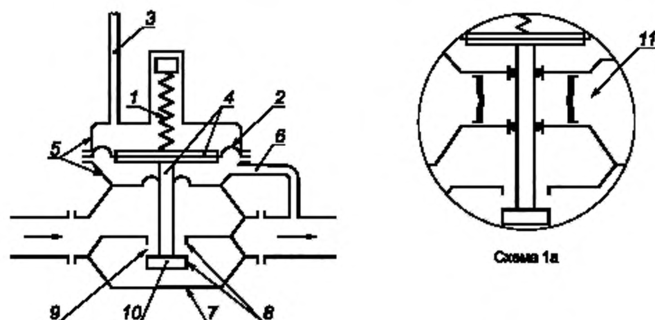
1 — элемент настройки; 2 — элемент измерения давления (1 и 2 — органы управления); 3 — салун (вентиляция/воздуховод); 4 — сервопривод; 5 — корпус сервопривода; 6 — импульсная трубка; 7 — корпус регулятора; 8 — седла клапана; 9 — кольцо седла клапана; 10 — регулирующий элемент; 11 — схема 1а
