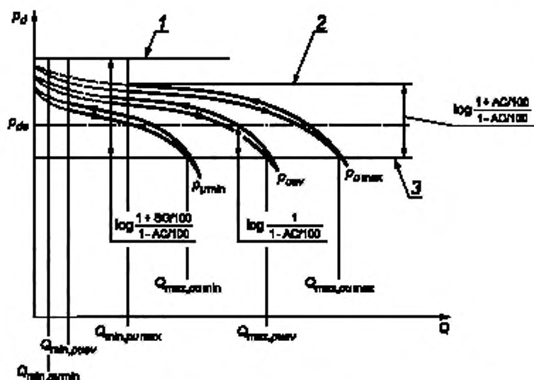
1 — максимальный предел для p_d ; 2 — максимальный предел для p_d с объемным расходом Q вне зоны байпасов; 3 — минимальный предел для p_d
