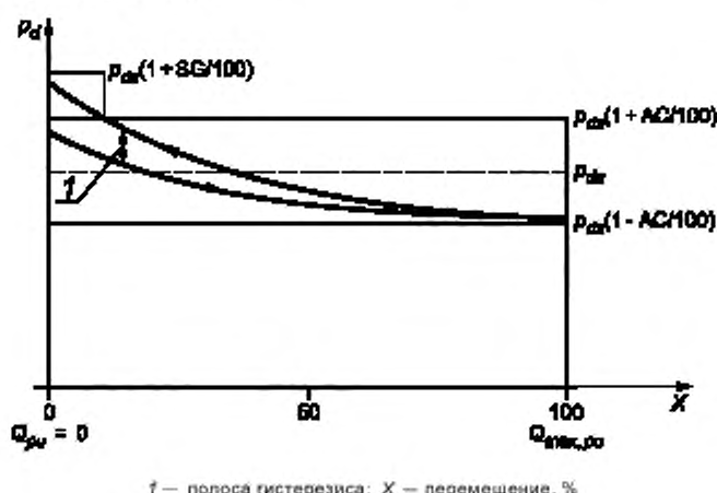
Рисунок Б.1 — График выходного давления, соответствующий разным позициям элемента управления регулятора прямого действия
