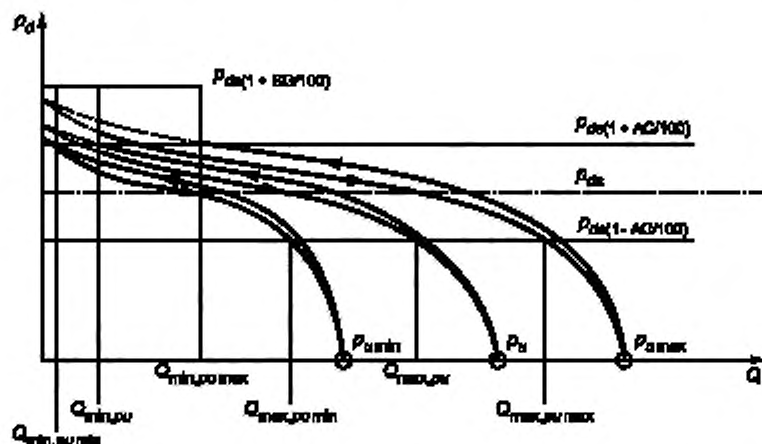
Рисунок 5 — Набор характеристик для изображения наивысших объемных расходов с гарантированной точностью и низших объемных расходов ( p_{\text{де}} — постоянная величина, стабильные условия)
