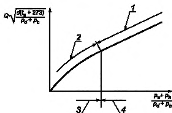
1 — линейный участок; 2 — нелинейный участок; 3 — докритическое поведение; 4 — критическое поведение
