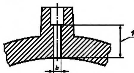
Рисунок 14 — Отвод давления
