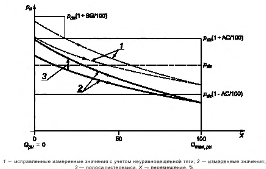
Рисунок Б.2 — График выходного давления, нанесенный на разные положения элемента управления в неутрансформированном регуляторе прямого действия
