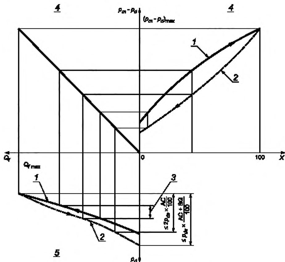
1 — открытие; 2 — закрытие; 3 — полоса гистерезиса; 4 — регулятор; 5 — пилот; X — диапазон перемещения, %
