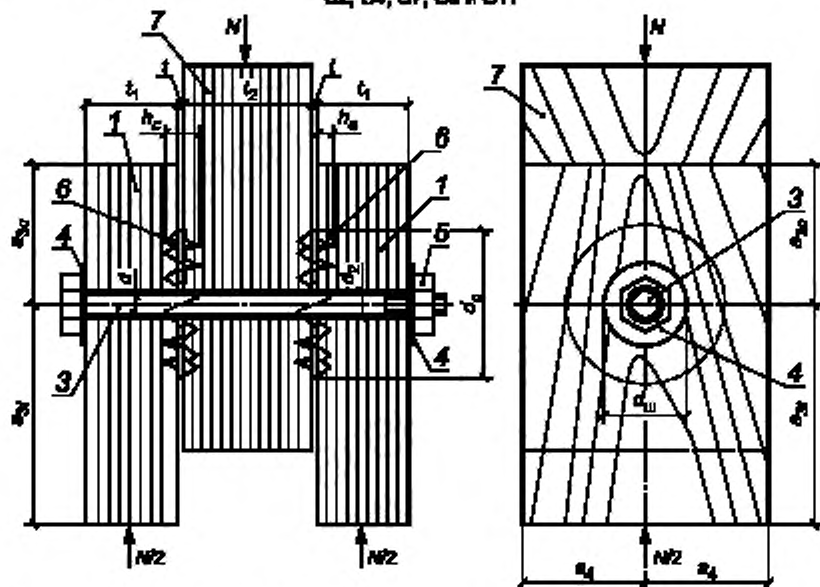
б) Схемы образцов двухсрезных соединений с двухсторонними зубчатыми шпонками типов С1, С5, С6, С8 и С10
