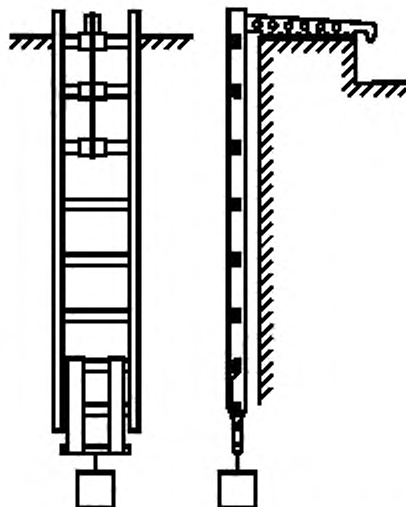
Рисунок 10 — Схема испытаний штурмовой лестницы в рабочем положении на прочность
