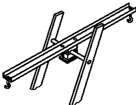
Рисунок 7 — Приспособление для испытания ступеньки на кручение
