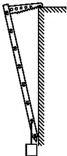
Рисунок 11 — Схема испытания крюка штурмовой лестницы на прочность
