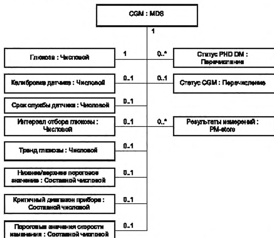
Рисунок 2 — Информационная модель предметной области глюкометра непрерывного действия
