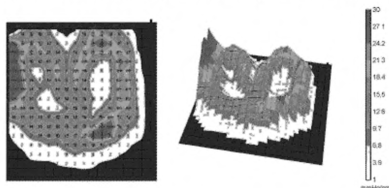
Рисунок 5 — Контур градиента и изображение поверхности для графика давления на рисунке 3 и рисунке 4
