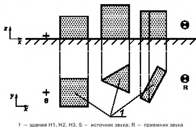
Рисунок 27 — Три экранирующих здания (N1, N2, N3) между источником и приемником
