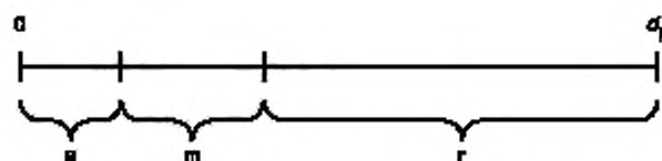
Рисунок 6 — Зоны распространения звука согласно ИСО 9613-2 (рисунок 1)
