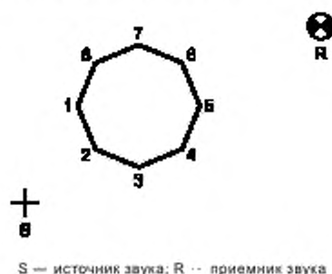
Рисунок 25 — Плоская поверхность с однородными акустическими свойствами и здание призматической формы, приемник на большой высоте
