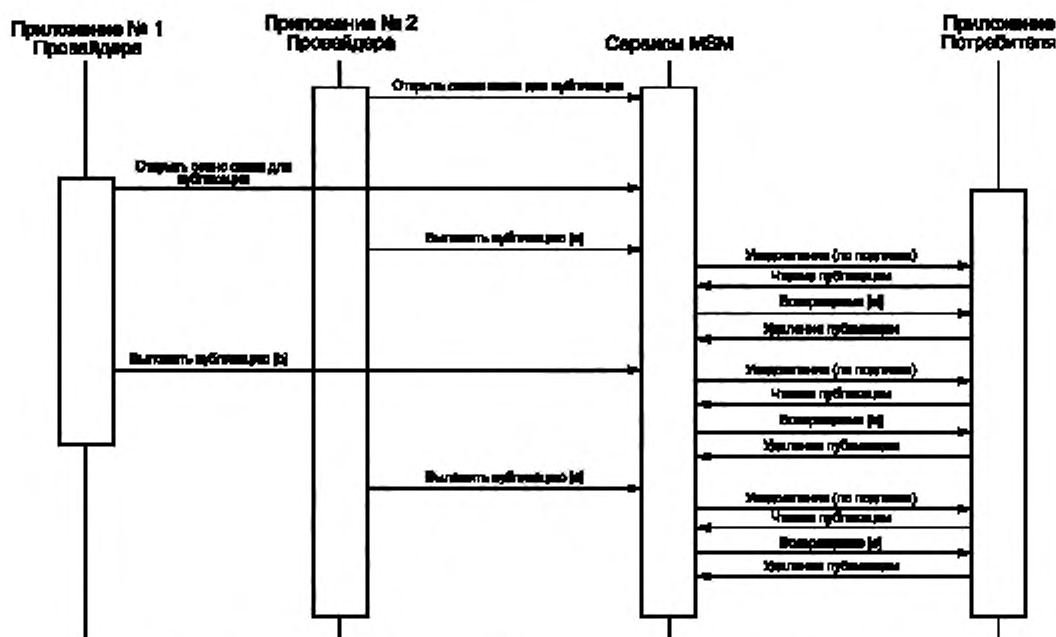
Рисунок 13 — Сценарий публикации с несколькими приложениями провайдера
