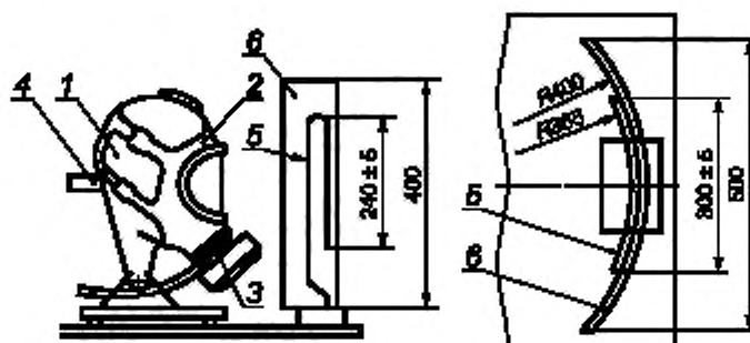
1 — металлический муляж головы человека; 2 — лицевая часть; 3 — легочный автомат; 4 — патрубок для подключения насоса «искусственные легкие»; 5 — источник теплового излучения; 6 — рефлектор
