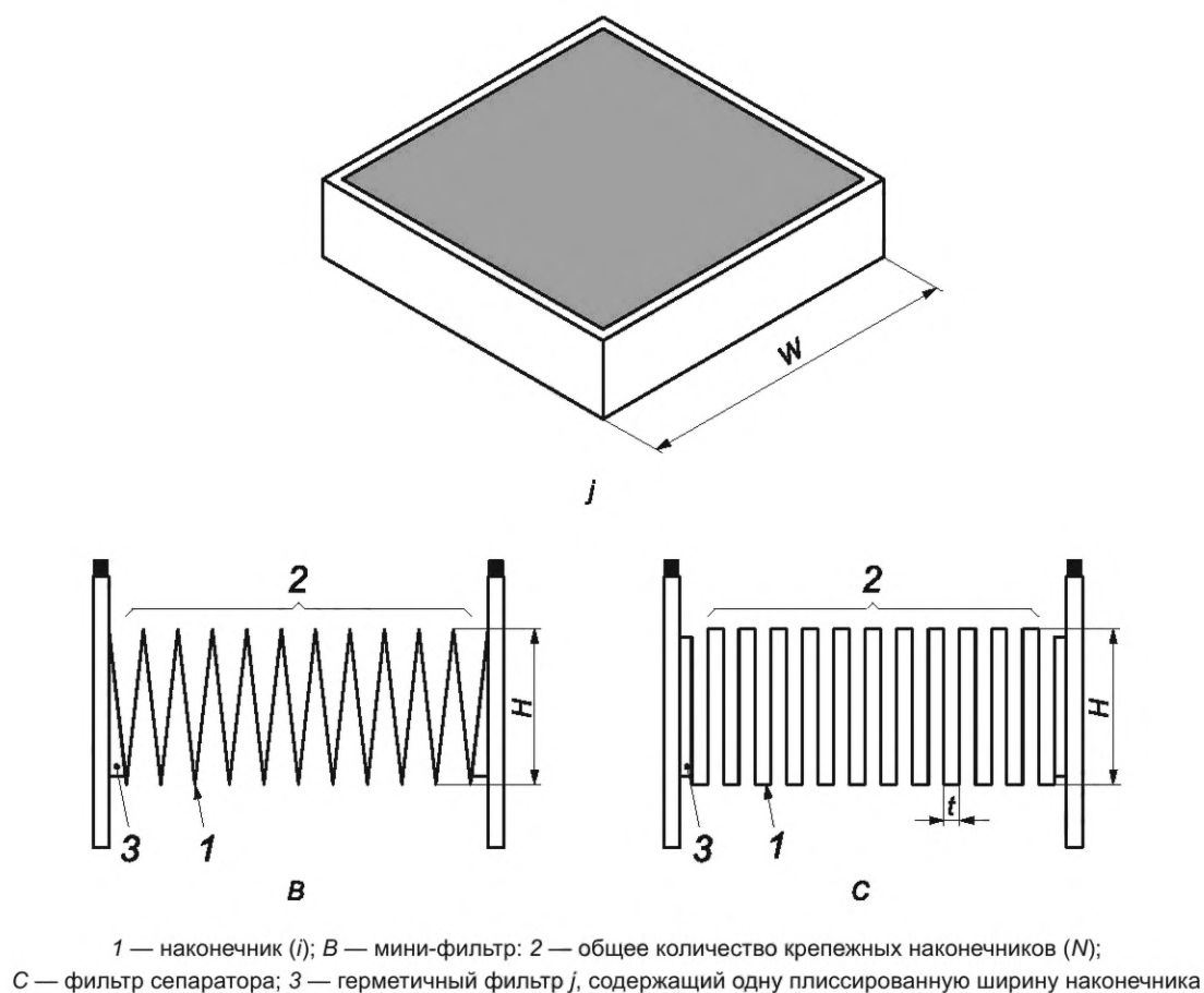
Рисунок Е.4 — Гофрированный фильтр с одним пакетом. Оценка чистой площади фильтрации
