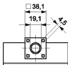
а) Пылеулавливающая трубка
