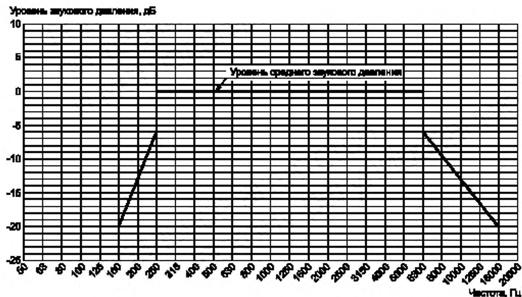
Рисунок А.2 — Поле допусков частотной характеристики для носимого тифлофлешплеера
