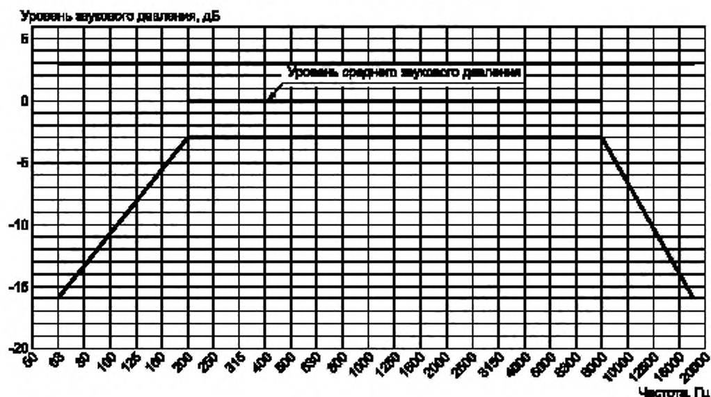
Рисунок А.1 — Поле допусков частотной характеристики для переносного тифлофлешплеера
