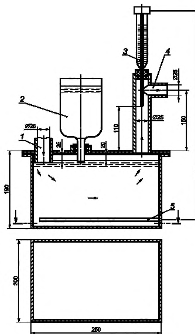
1 — штуцер для подключения насоса «искусственные листья»; 2 — пополняющий резервуар; 3 — терморегулирующее устройство; 4 — штуцер для подключения тройника; 5 — электронагреватель
