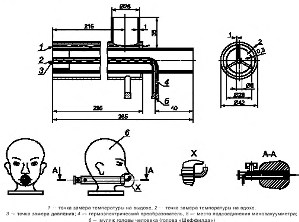
Рисунок 5 — Муляж головы человека (голова «Шеффилда»)
