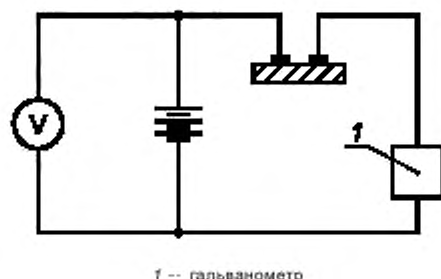
Рисунок Б.1 — Электрическая схема измерения тока микроамперметром или гальванометром
