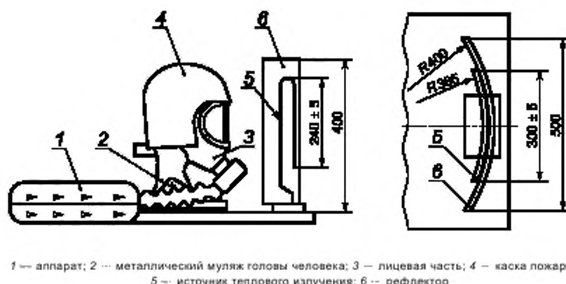
Рисунок 4 — Схема установки по определению устойчивости к воздействию теплового потока
