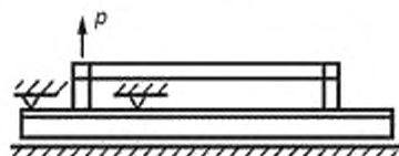
Рисунок 9 — Схема определения прочности соединения стоек правил и полутерков с основанием
