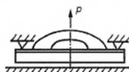
Рисунок 10 — Схема определения прочности соединения ручек терок с основанием и определения прочности конструкции цельнолитых терок и полутерков
