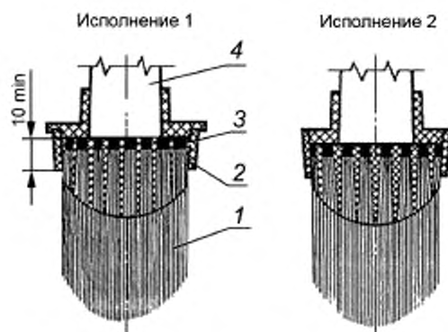
Рисунок А.2 — Исполнения кистей-ручников типа КРС. Исполнения 1, 2
