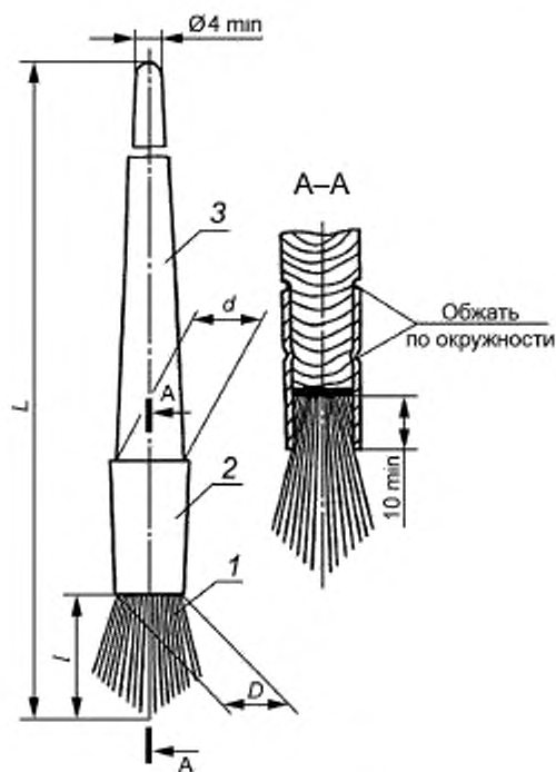
Рисунок 10 — Кисть филоночная типа КФК. Исполнение 1
