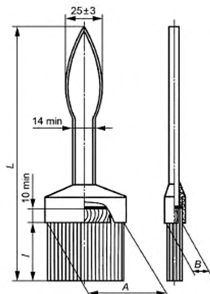
Рисунок 9 — Кисть флейцевая типа КФ. Исполнение 2
