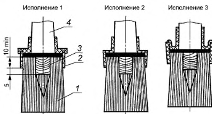
Рисунок А.1 — Исполнения кистей-ручников типов КР, КРО. Исполнения 1—3
