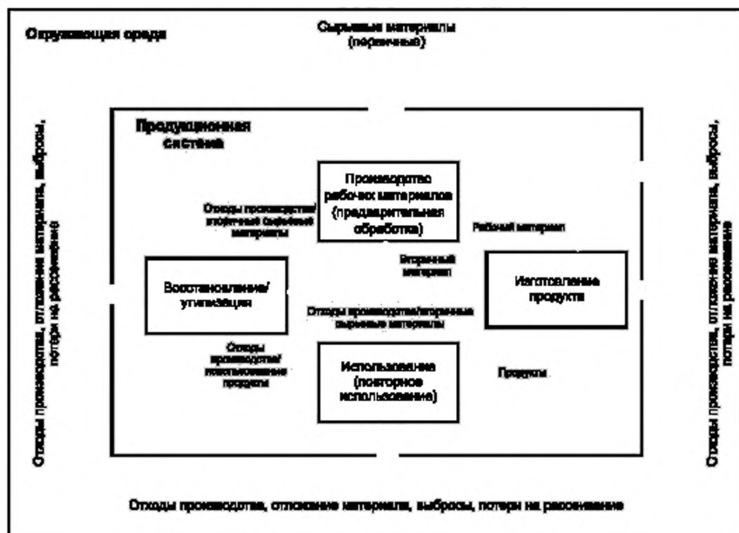
Рисунок 3 — Расход ресурса и движение материалов в течение жизненного цикла
