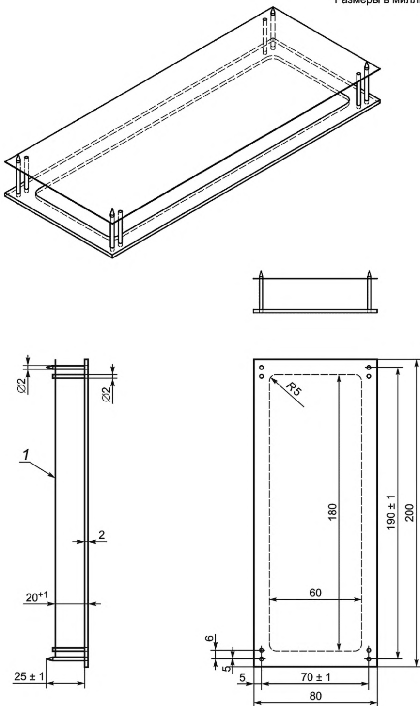
b) Держатель испытуемого образца для процедуры В
