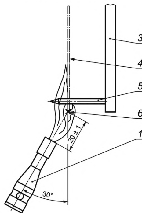
д) Воспламенение нижней кромки
