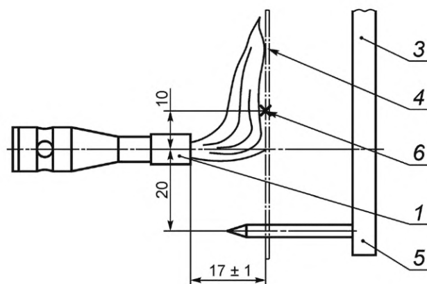
а) Воспламенение поверхности
