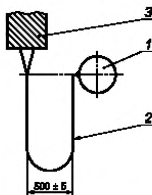
1 — контрольный груз; 2 — свободная петля испытываемого образца; 3 — опора
