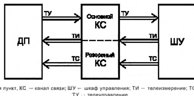
Рисунок 9 — Передача команд телеуправления и сигналов в диспетчерский пункт
