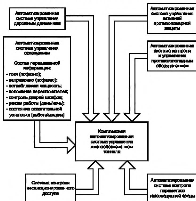
Рисунок В.1 — Схема информационного обмена АСУ освещением в составе комплексной автоматизированной системы управления жизнеобеспечением тоннеля
