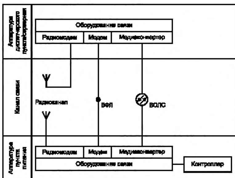
Рисунок 6 — Схема комбинированных каналов связи
