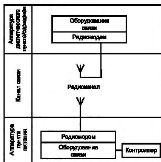
Рисунок 5 — Схема беспроводного канала связи
