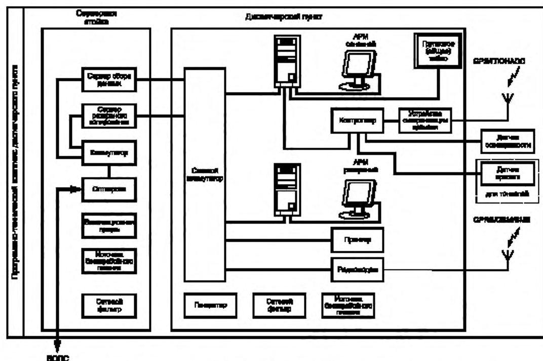
Рисунок 2 — Типовая структура диспетчерского пункта АСУ освещением
