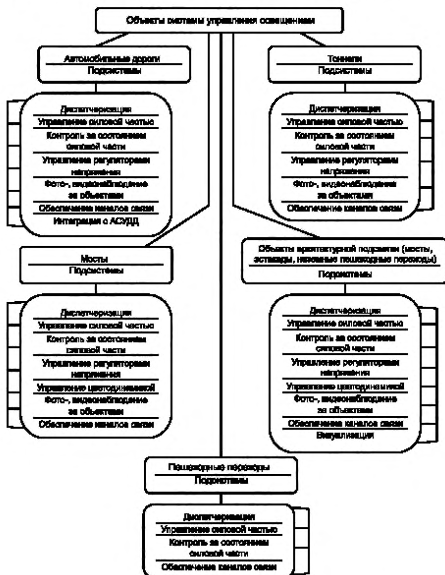
Рисунок Г.1 — Объекты и подсистемы, входящие в систему управления освещением
