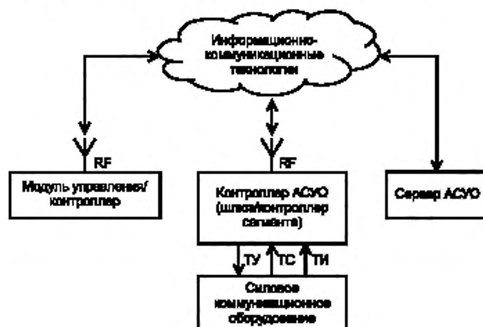
Рисунок Б.5 — Обмен информацией по беспроводным радиоканалам RF через «облачные» информационно-коммуникационные технологии
