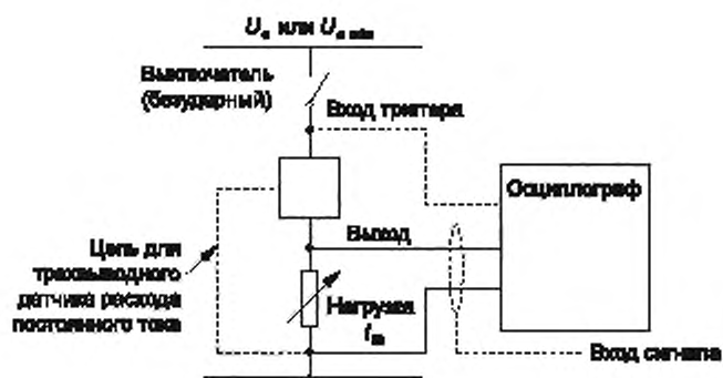
Рисунок 3 — Испытательная цепь для проверки задержки готовности
