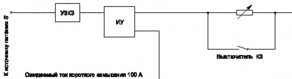
Рисунок 6 — Испытание на короткое замыкание
