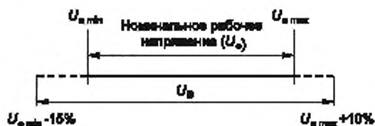
Рисунок 2 — Взаимосвязь между U_e и U_B
