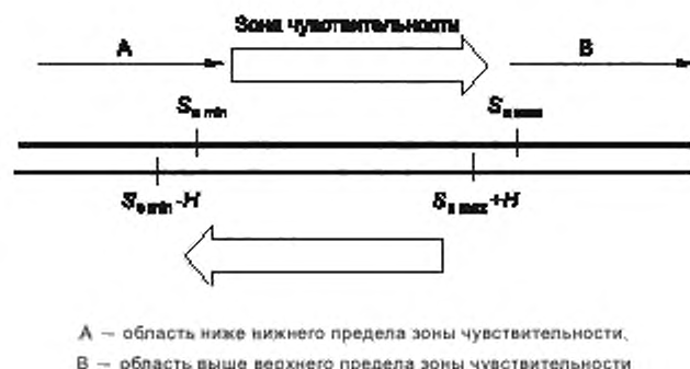
Рисунок 1 — Взаимосвязь между рабочими точками датчика расхода
