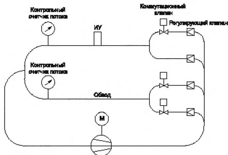
Рисунок 7 — Испытание заданной точки и задержек времени
