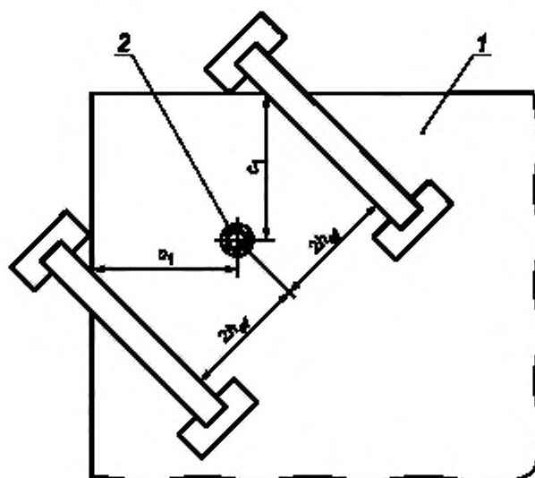
1 — строительное основание; 2 — испытуемый анкер
