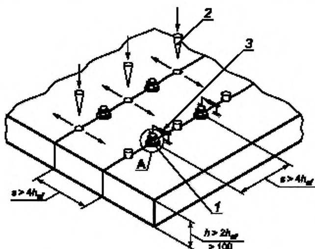
1 — анкер; 2 — клин; 3 — индикатор измерения ширины раскрытия трещины
