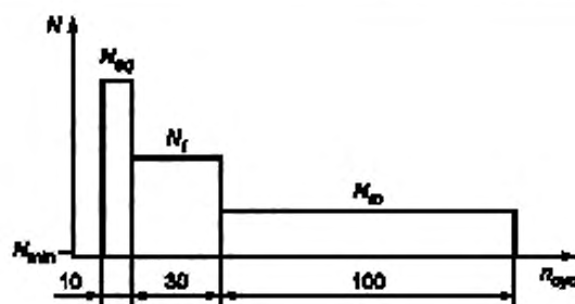
Рисунок 7.10 — Циклограмма испытаний для серии К2
