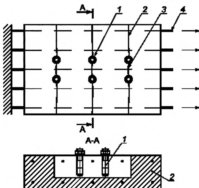
1 — анкер; 2 — инициатор трещины; 3 — трещины; 4 — арматура
