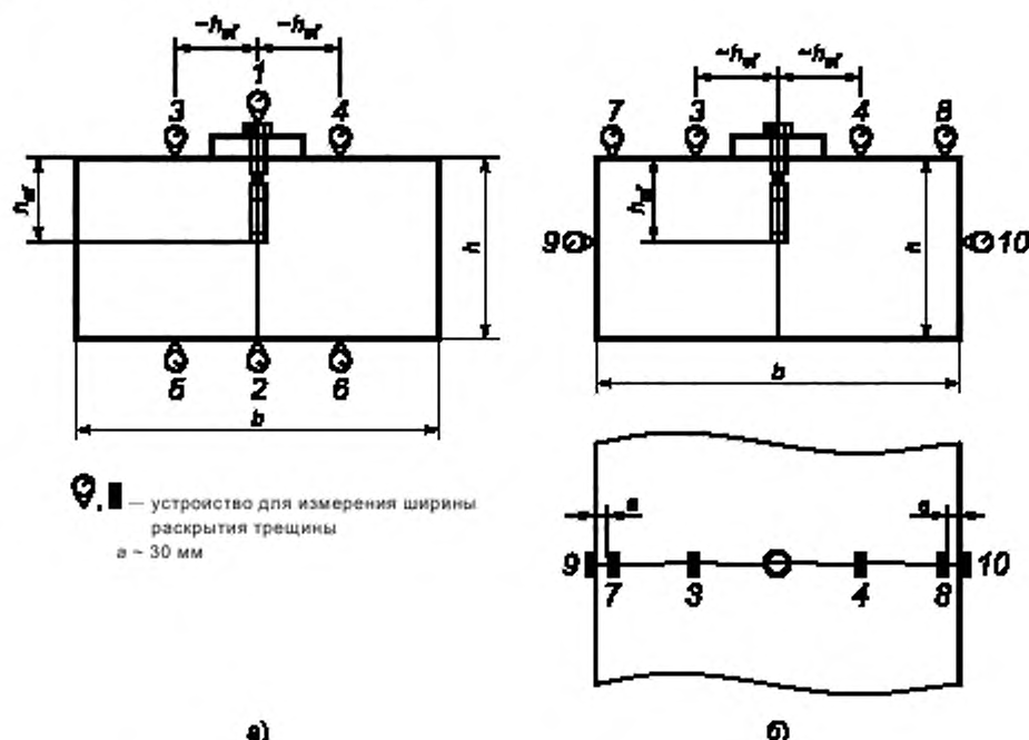
Рисунок 7.3 — Измерения по определению ширины раскрытия трещины
