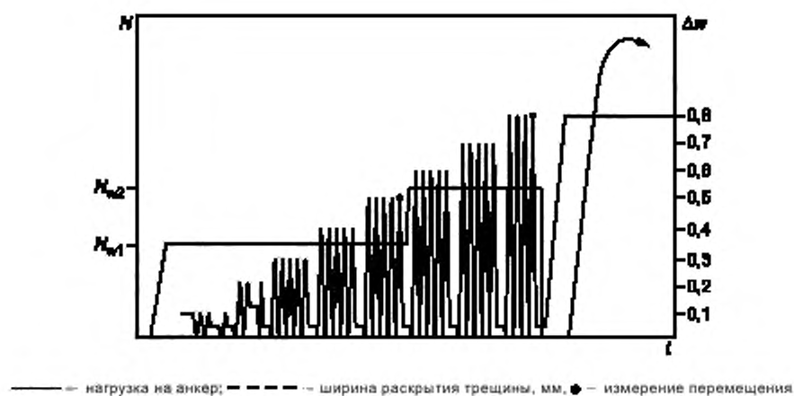
Рисунок 7.15 — Циклограмма испытаний анкерного крепежа
