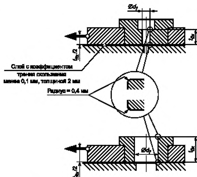
Рисунок 7.5 — Пример оснастки для испытания на сдвиг
