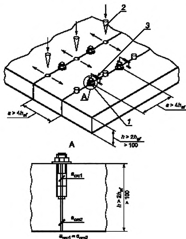
1 — анкер; 2 — клин; 3 — индикатор измерения ширины раскрытия трещины
