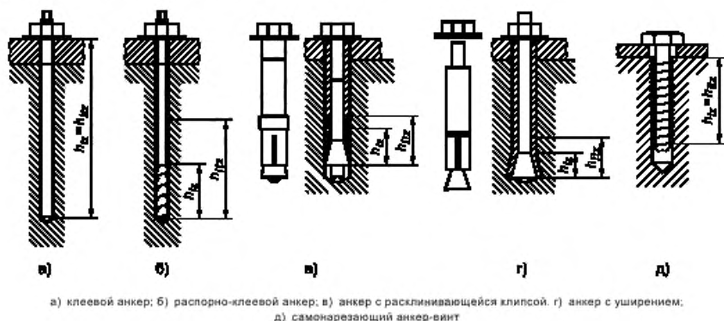
Рисунок 7.4 — Зона эффективного восприятия нагрузки, h_{Rz}
