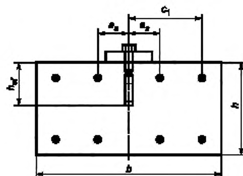
a_s — расстояние между осями анкера и арматурного стержня; b — ширина строительного основания; c_1 — расстояние от оси анкера до края строительного основания; h — толщина строительного основания; h_{af} — глубина анкерования
