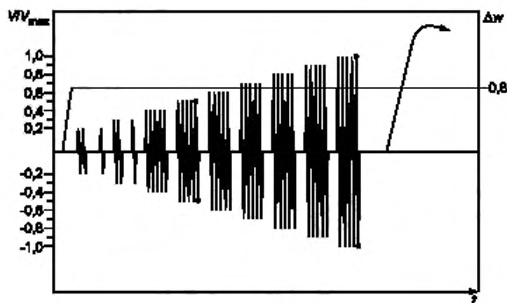
Рисунок 7.12 — Циклограмма испытаний анкерного крепежа на сдвиг
