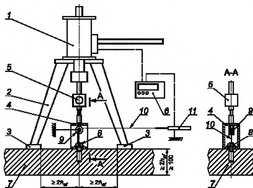
1 — домкрат с датчиком усилия (давления); 2 — силовая рама; 3 — опора силовой рамы; 4 — универсальное захватывающее устройство с тягой; 5 — шарнир; 6 — устройство регистрации контрольных параметров (силы, перемещения); 7 — строительное основание; 8 — испытуемый анкер; 9 — направляющий блок на независимом штативе; 10 — тонкая проволока; 11 — индикатор перемещения на независимом штативе
