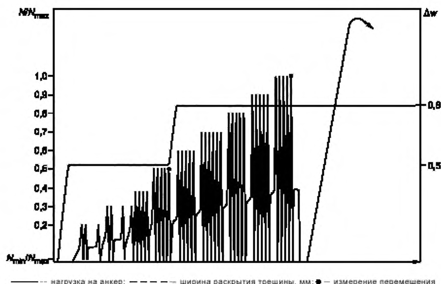
Рисунок 7.9 — Циклограмма испытаний анкерного крепежа на вырыв
