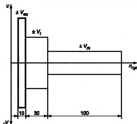
Рисунок 7.13 — Циклограмма испытаний для серии К2
