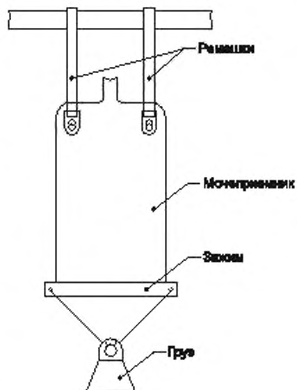
Рисунок 4 — Схема испытания на определение прочности системы крепления моче-приемников с пуговицами и петлями
