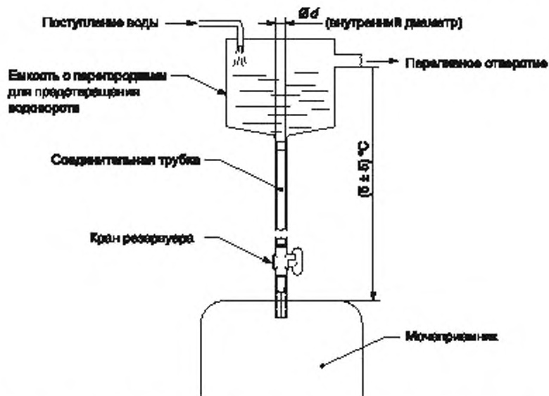
Рисунок 1 — Система заливки воды для определения испытательного объема
