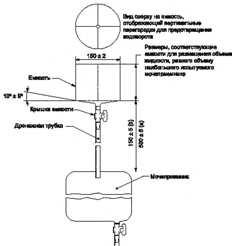
Рисунок 2 — Система заливки воды для испытания на отсутствие протекания (a) и измерения скорости наполнения (b)
