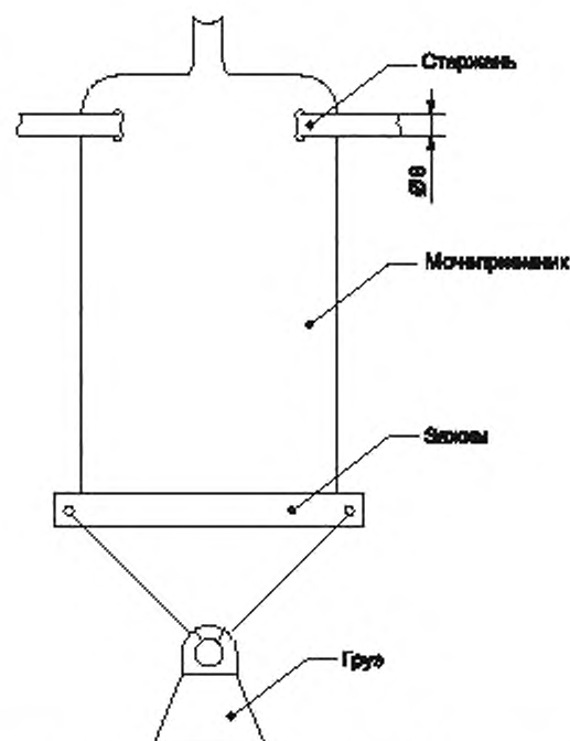
Рисунок 3 — Схема испытания на определение прочности системы крепления мочеприемников с прорезями
