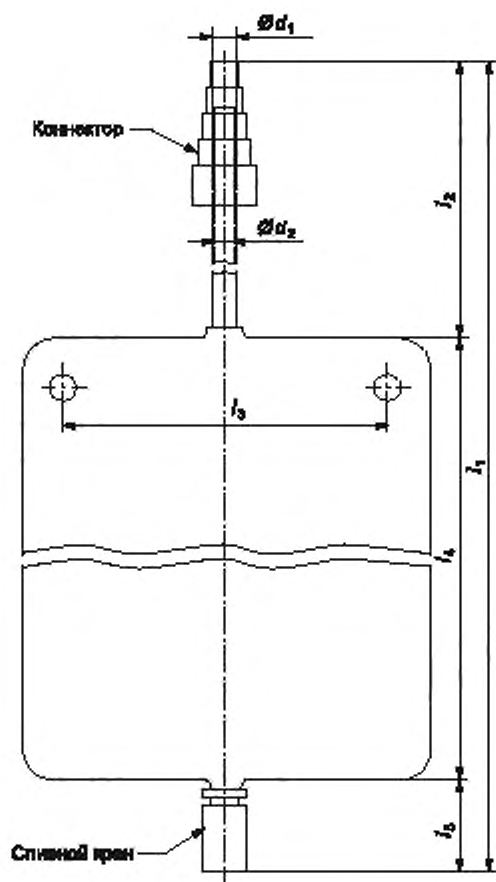
Рисунок А.1 — Стандартные размеры монеприемника
