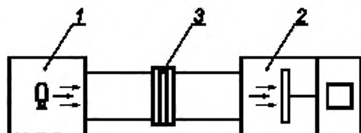
Рисунок А.5 — Схема поверки ИК взвешенных (твердых) частиц АИС КВ с использованием тестового аэрозоля
