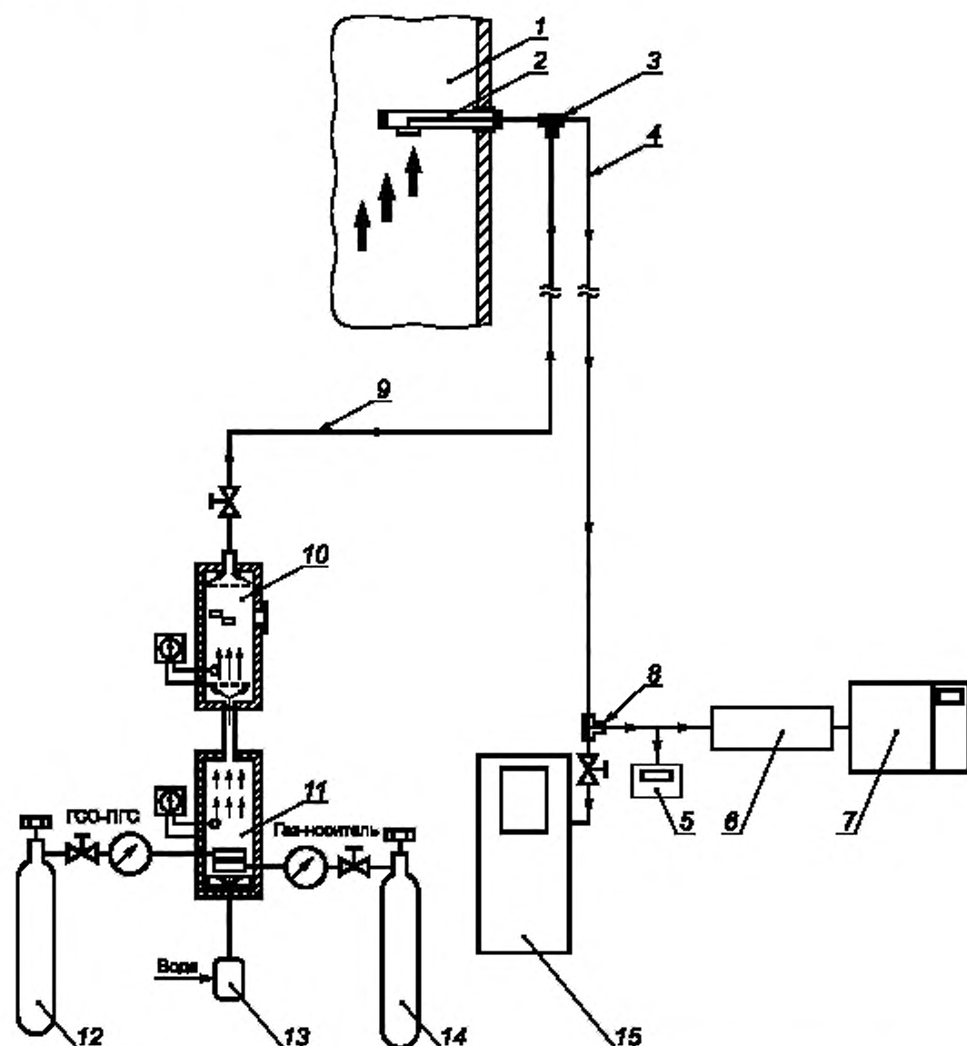
1 — газозод; 2 — зонд-пробоотборник АИС КВ; 3 — тройник-переключатель; 4 — трубопровод транспортировки пробы АИС КВ; 5 — аналитический блок для определения влажности (для АИС КВ с предварительным удалением паров воды при подготовке пробы); 6 — система подготовки пробы АИС КВ; 7 — газоаналитический блок АИС КВ; 8 — тройник; 9 — линия для транспортировки многокомпонентной увлажненной ГС на основе ГСО-ПГС; 10 — рабочая камера-смеситель; 11 — газовый генератор для получения многокомпонентной увлажненной ГС на основе ГСО-ПГС; 12 — баллон с многокомпонентной ГСО-ПГС; 13 — насос для подачи воды; 14 — баллон с газом-носителем — азотом; 15 — мобильный поверочный комплекс (с каналом определения влажности)
