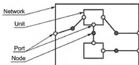
Рисунок 3 — Графическое представление объекта данных «модель системы сбора и подготовки»
