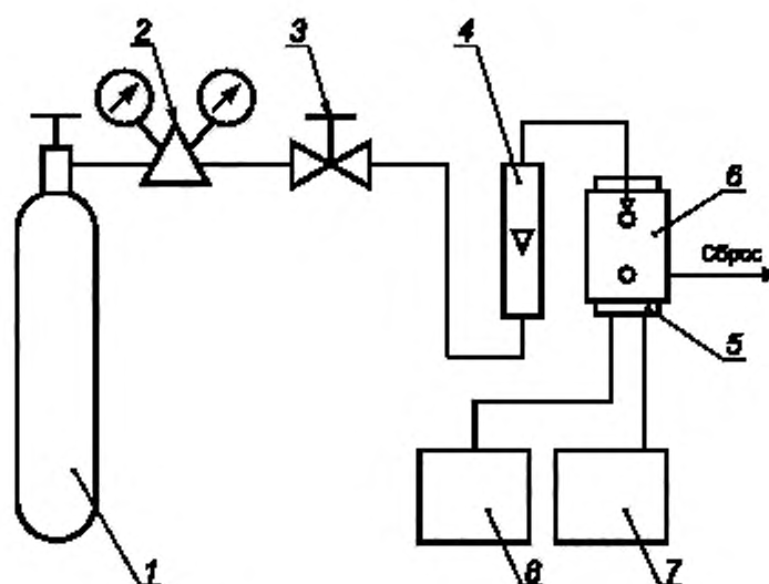
Схема подачи ГС на СИ при проведении поверки
