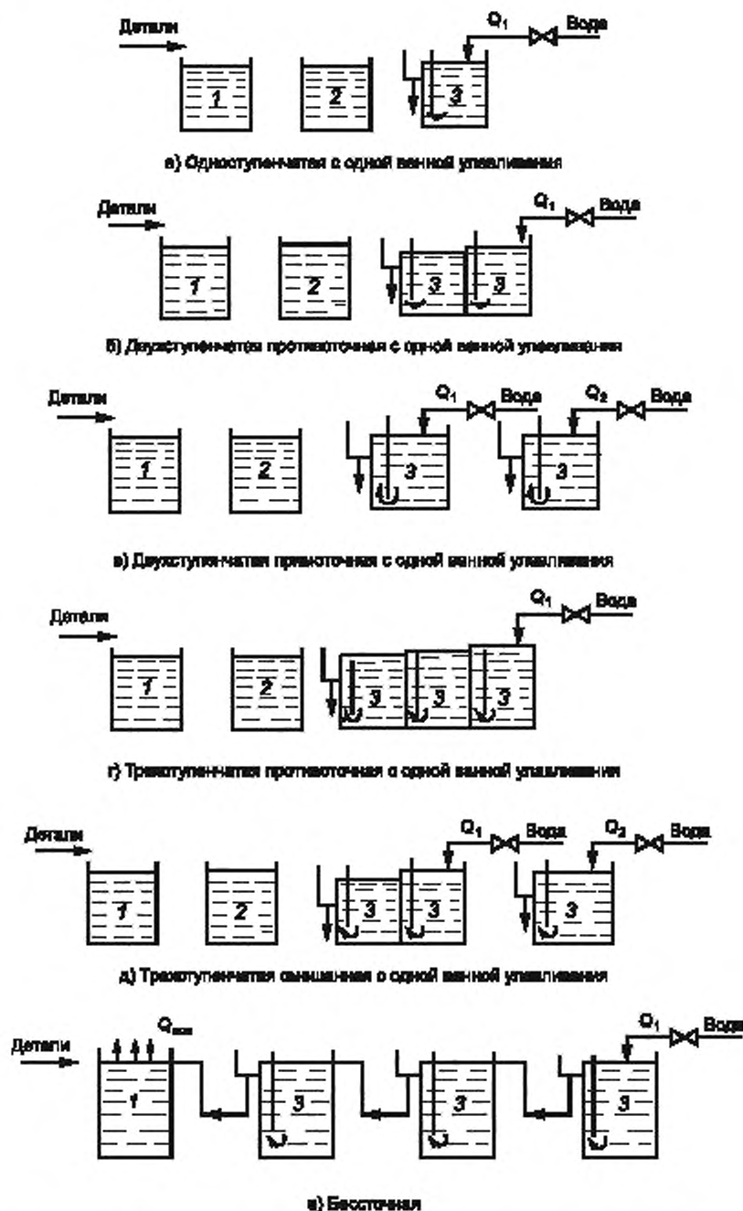
Рисунок 2 — Схемы промывок
