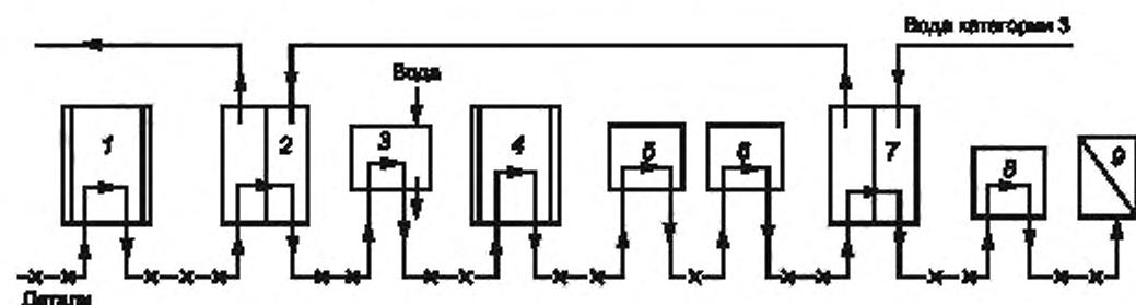
1 — ванна активации; 2, 7 — ванны промывки; 3 — ванна финишной промывки водой категории 3 (непроточная или циркулирующая); 4 — ванна нанесения покрытия драгметаллами; 5, 6 — ванны-уловители с водой категории 3; 8 — обдув сжатым воздухом или центрифугирование; 9 — термосушка
