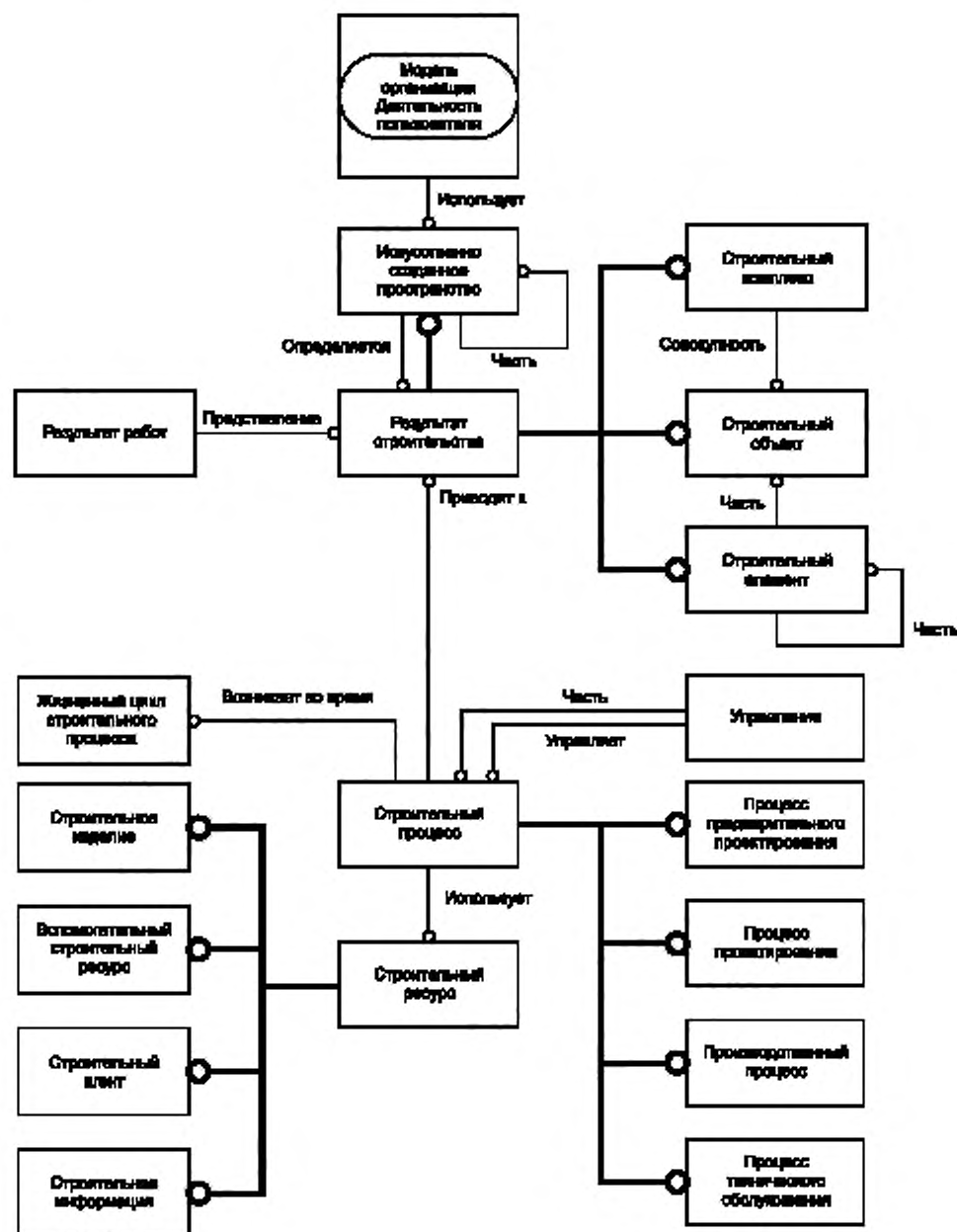
Рисунок 1 — Классы и их основные взаимосвязи
