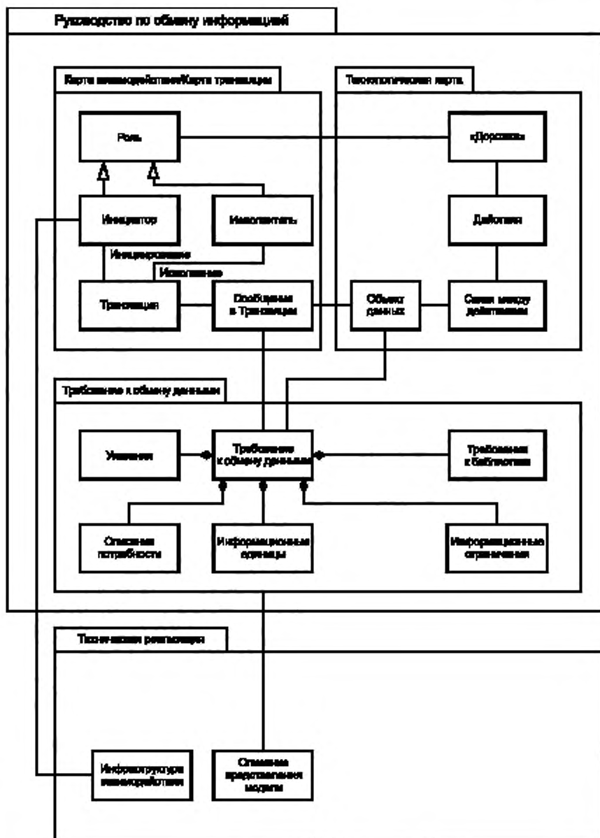
Рисунок 3 — Базовая инфраструктура IDM
