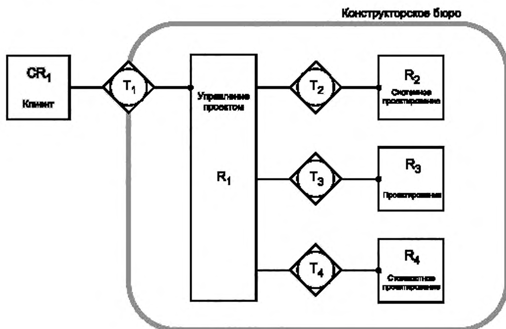
Рисунок В.2 — Карта взаимодействия
