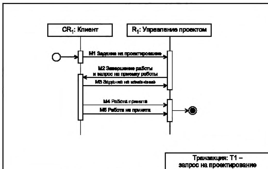
Рисунок В.3 — Карта транзакции
