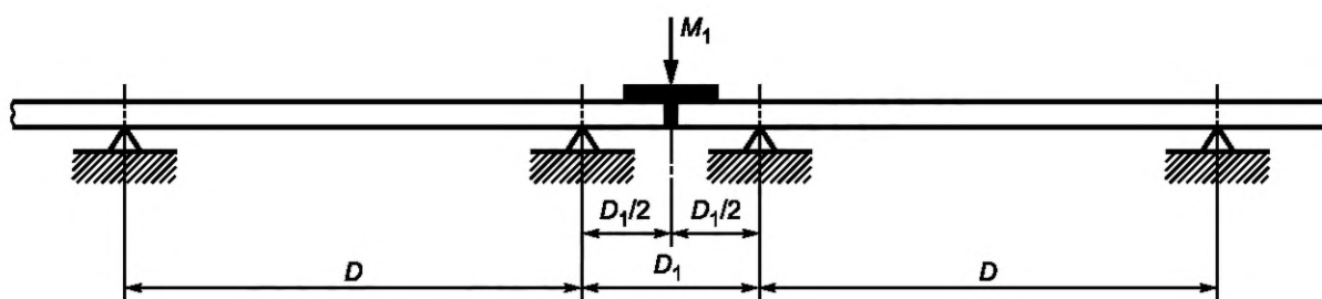
Рисунок 102 — Испытание соединения механической нагрузкой
