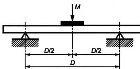
Рисунок 101 — Испытание механической нагрузкой прямого блока
