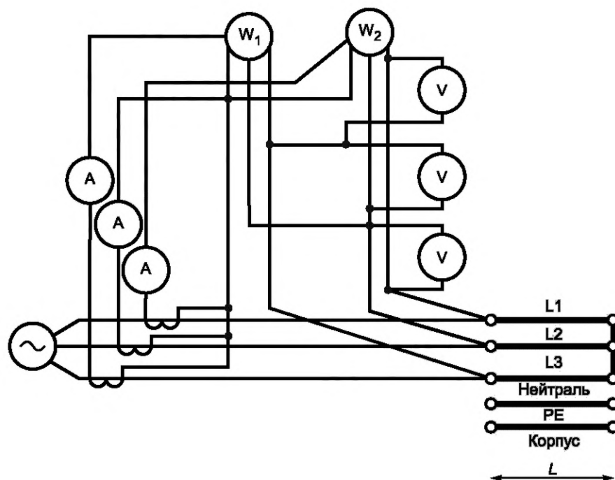
Рисунок ВВ.1 — Определение характеристик фазовых проводов
